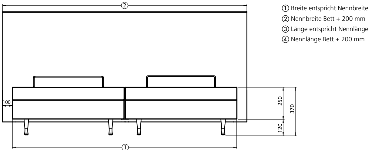
Frontansicht:
